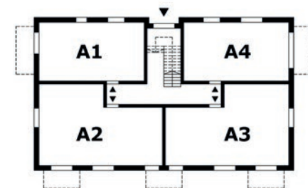
RZUT PARTERU
